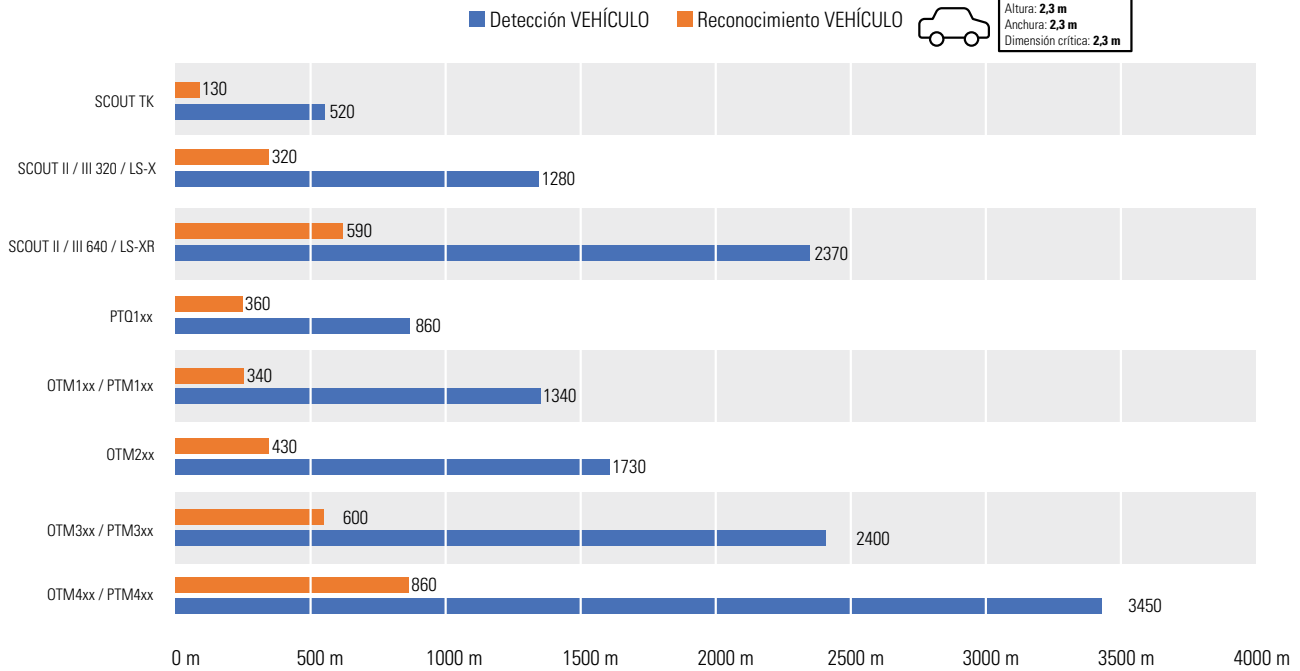
Rendimiento de la gama de productos: vehículo
