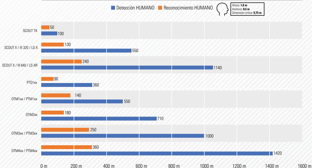
Rendimiento de la gama de productos: humano
