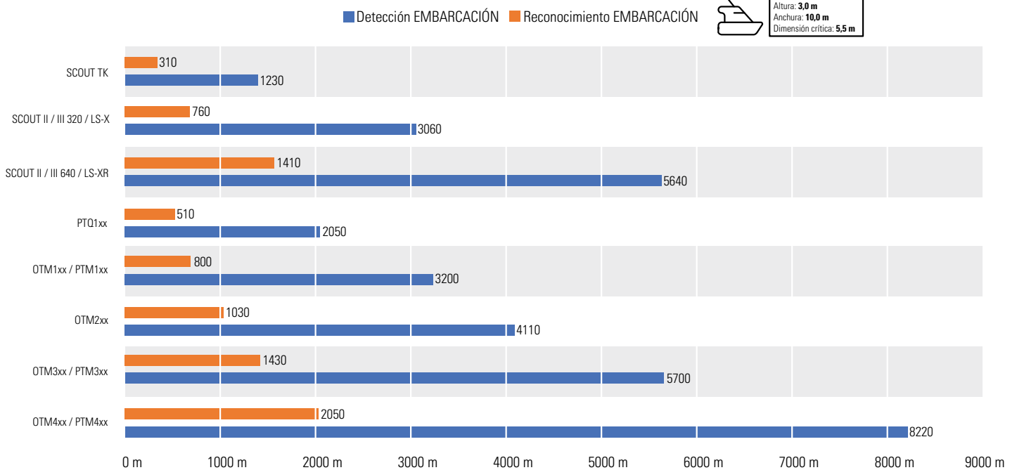
Rendimiento de la gama de productos: embarcación
